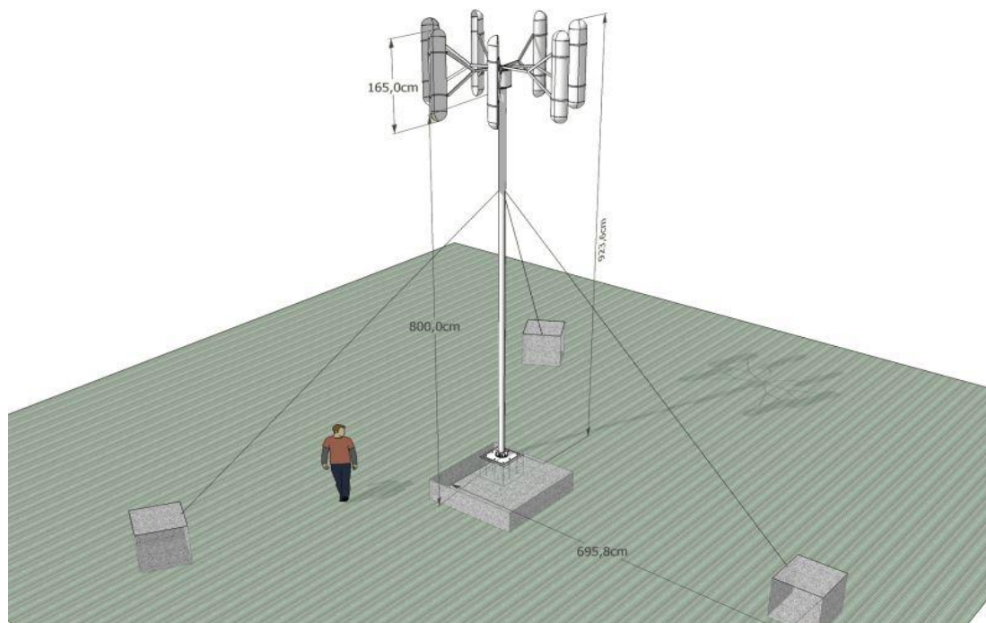
Rysunek 41. Parametry techniczne mikroturbiny wiatrowej (źródło: http://generatory-wiatrowe.pl/?page_id=21 )
